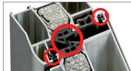
3 Dichtungsebenen garantieren optimalen Schutz gegen Wärmeverlust durch Zugluft
