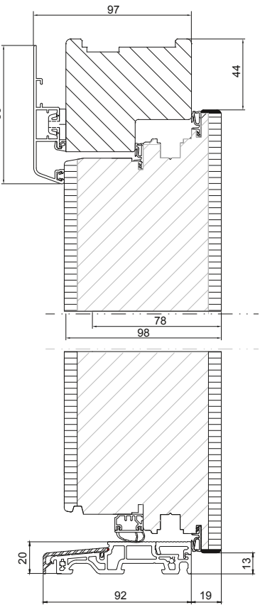
Holz-Alu Öko 98
