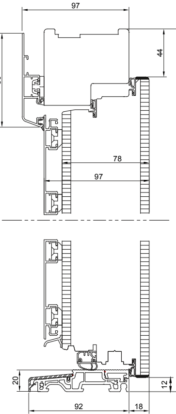
Holz-Alu Öko 78
